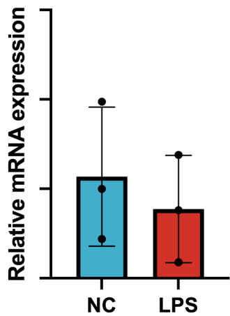
PTPRN
