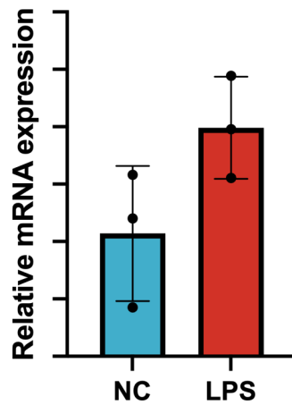
SYT1
