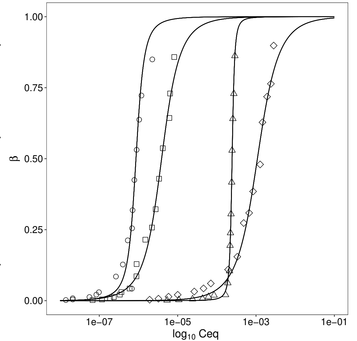
Zimm-Bragg model
