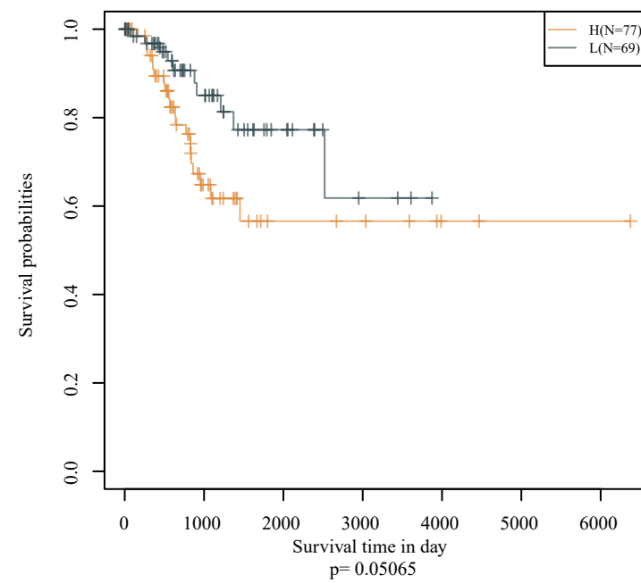
OPN3
