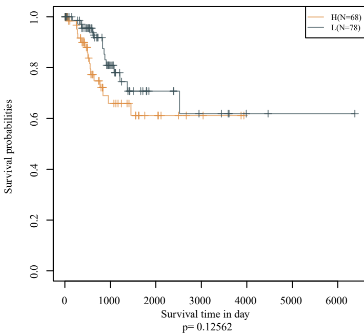
CXCL2
