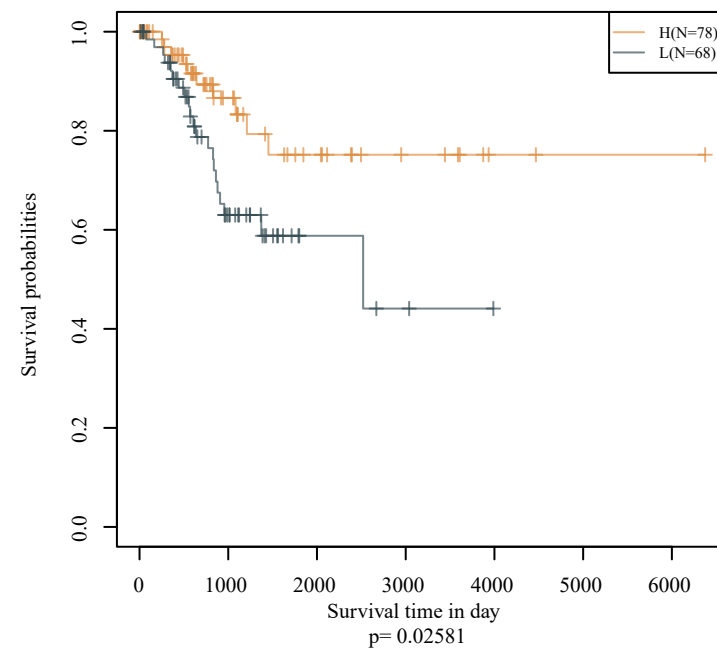
ASCL2
