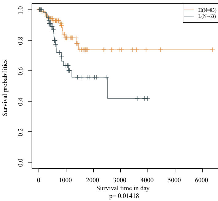
ALG1L
