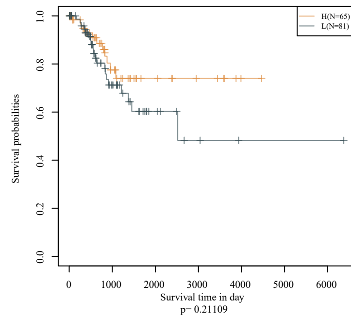
SERPINF1
