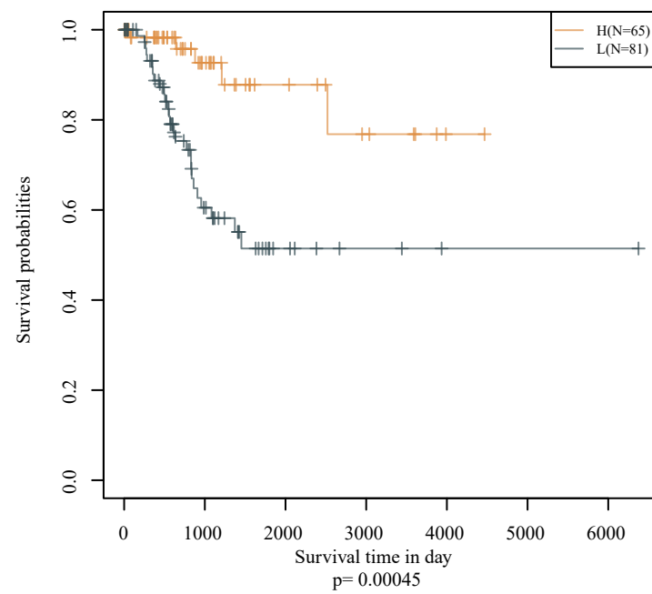
DES
