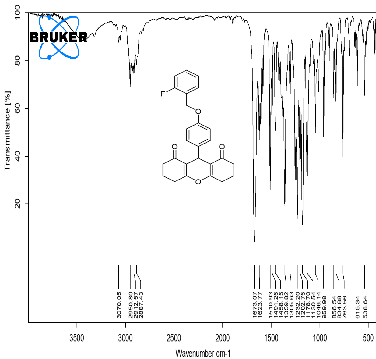
IR spectrum of 4e
