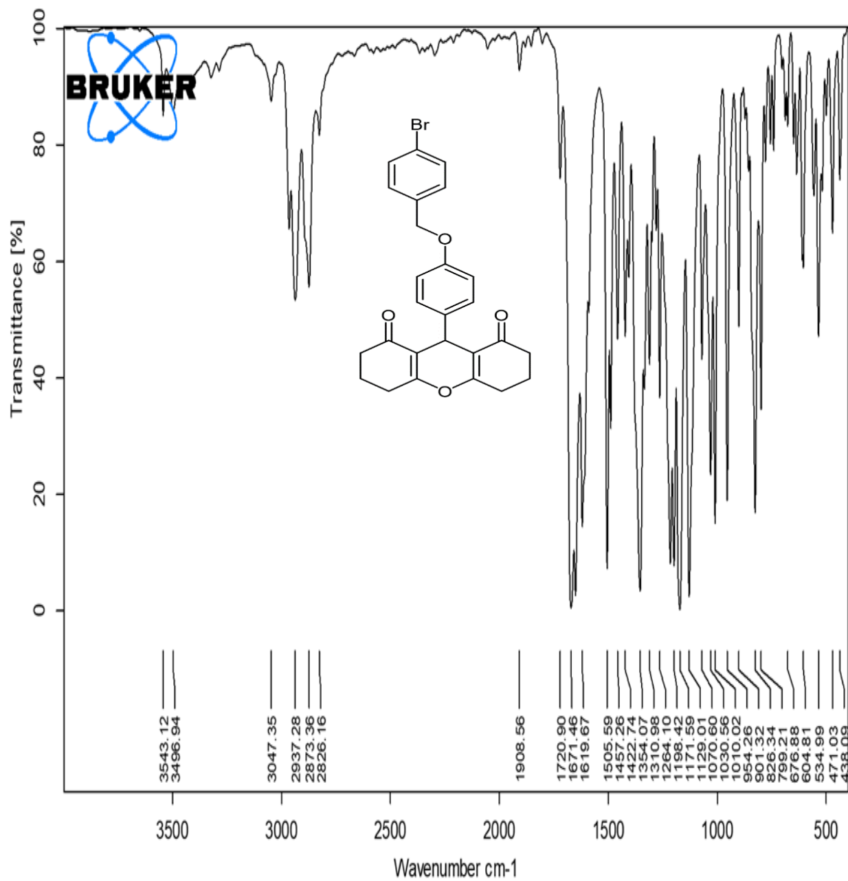
IR spectrum of 4b
