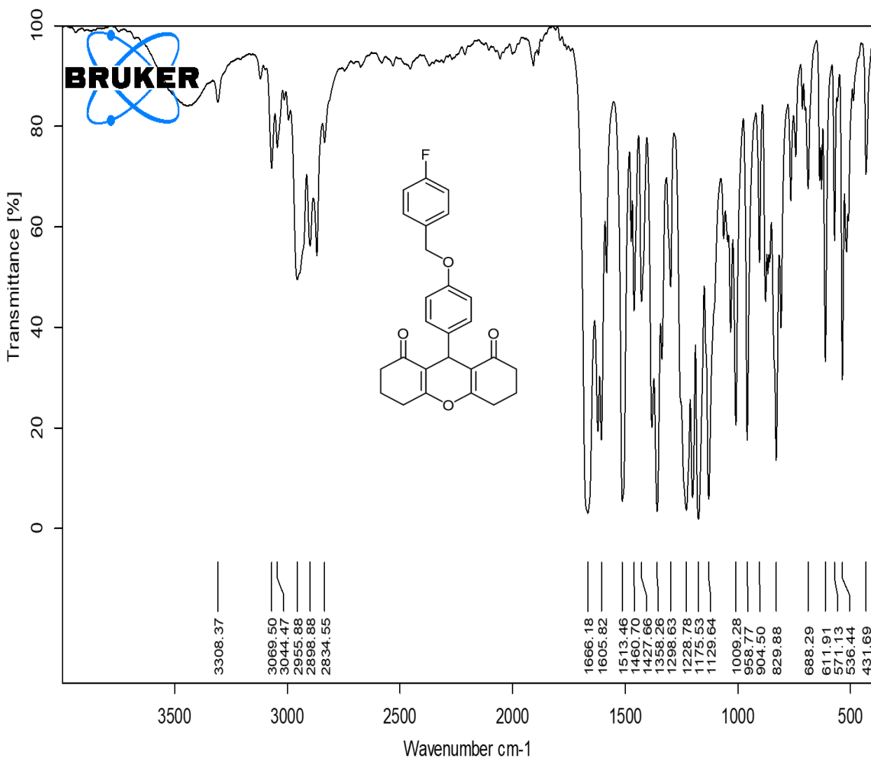
IR spectrum of 4d
