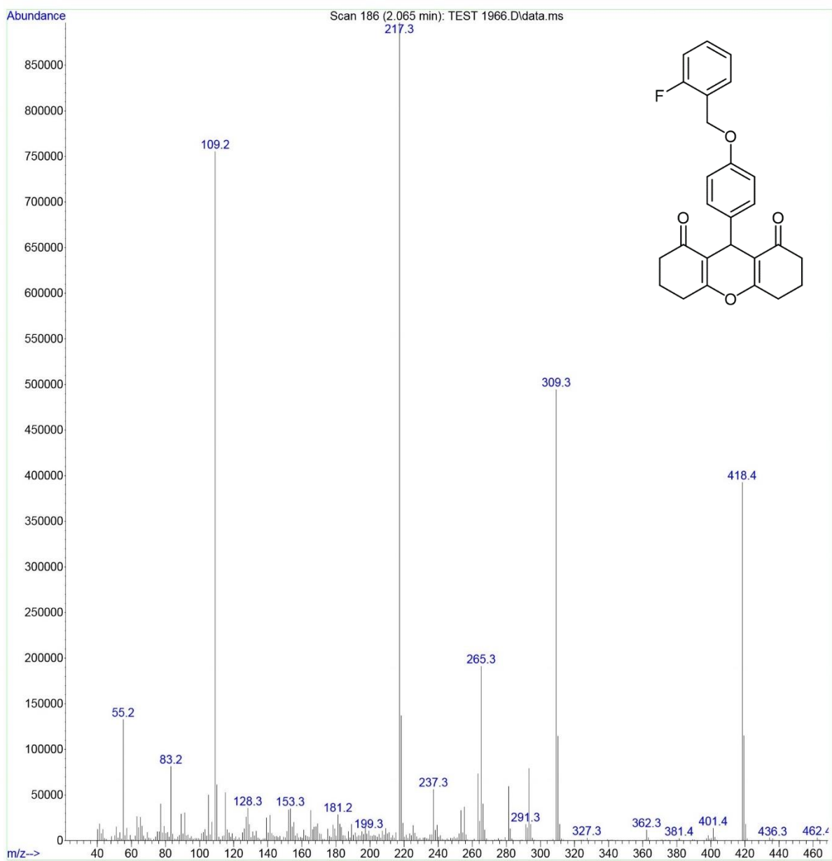
Mass spectrum of 4e
