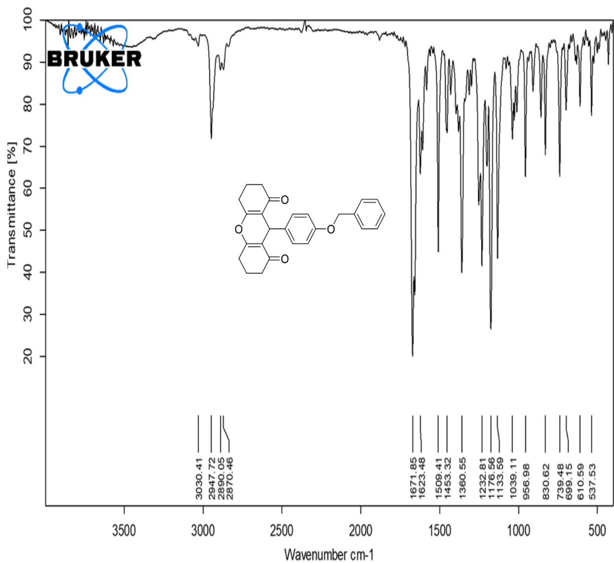
IR spectrum of 4a
