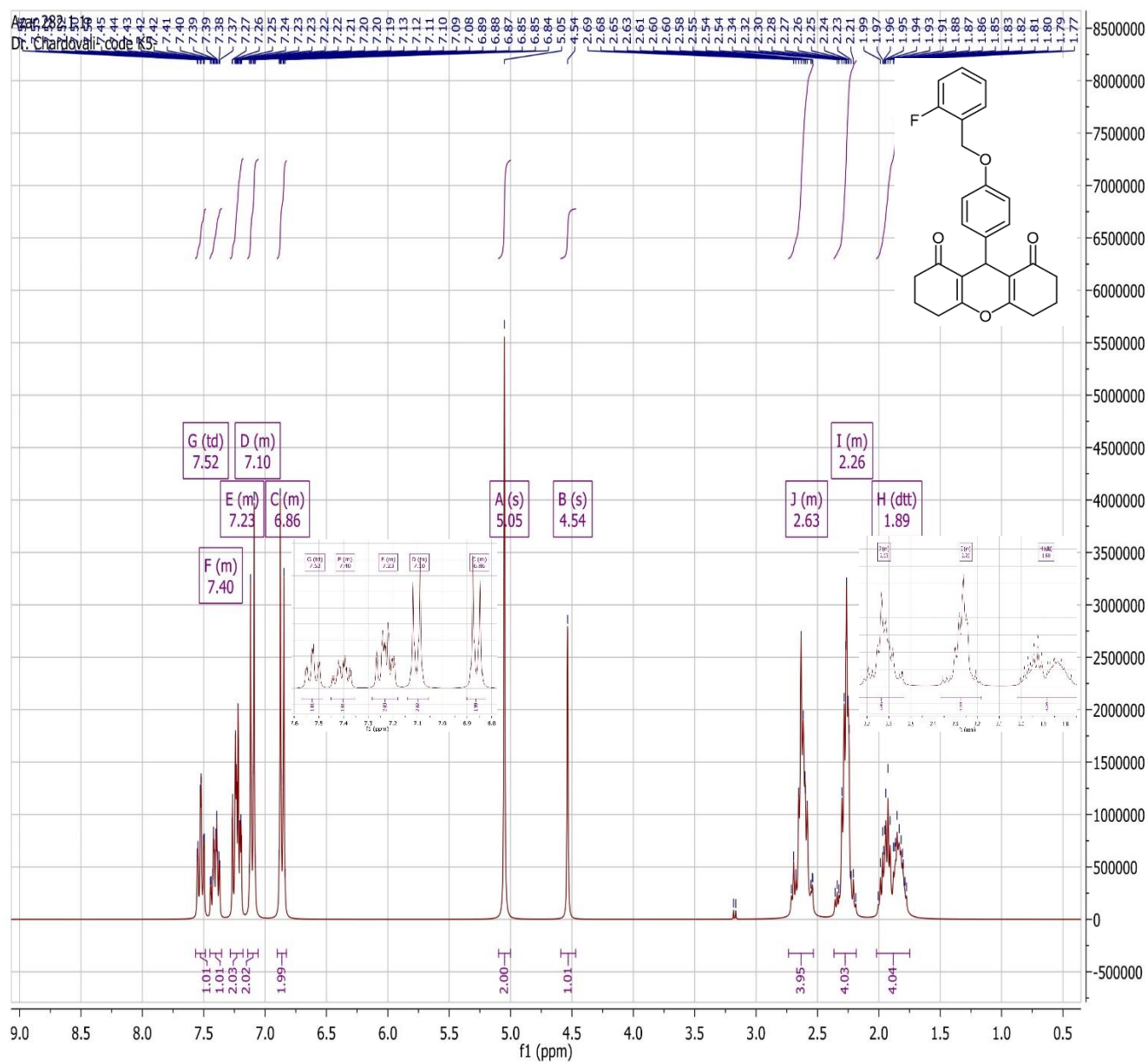
1 H-NMR spectrum of 4e
