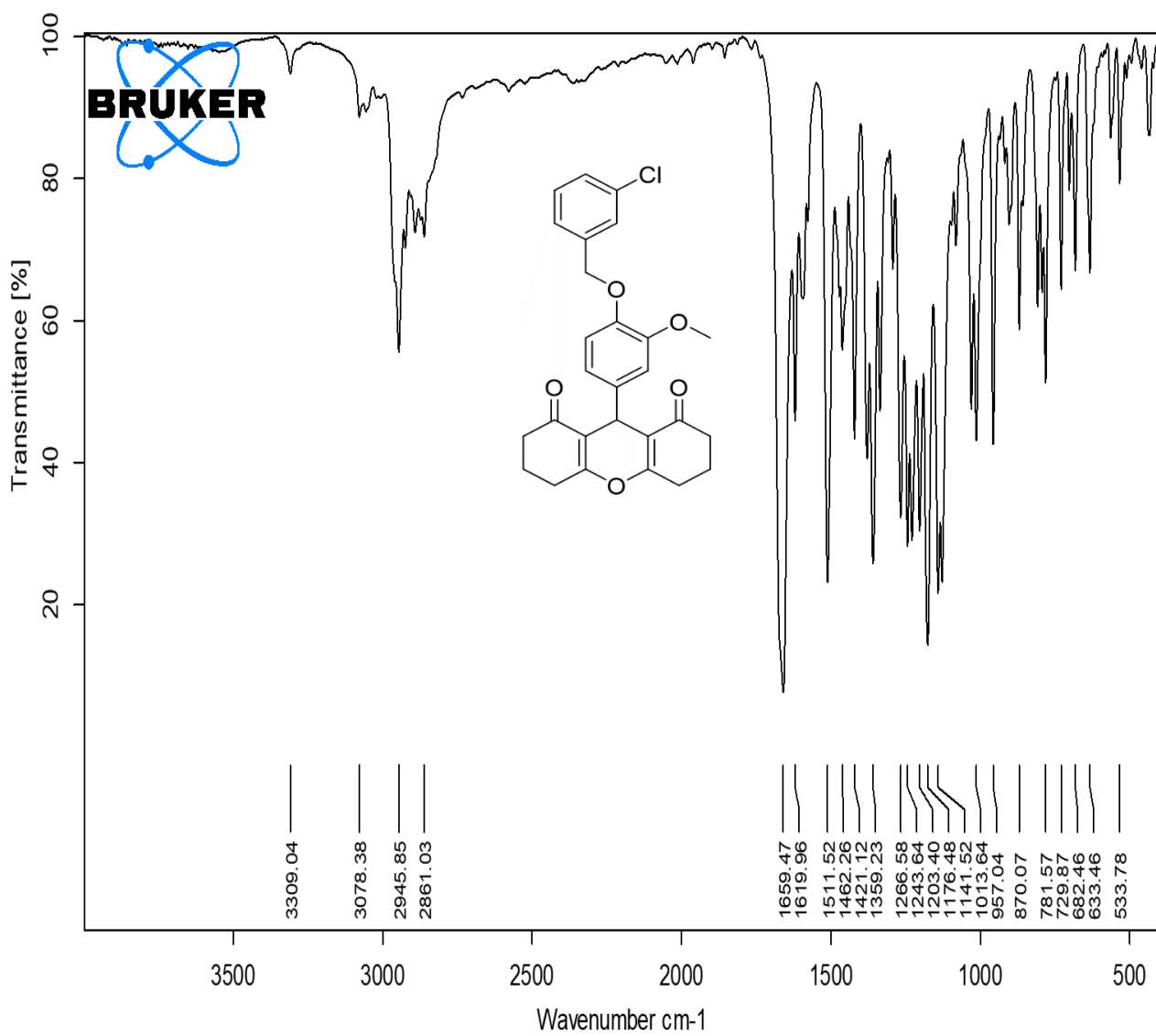
IR spectrum of 4k
